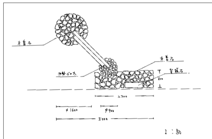
二班 図面
